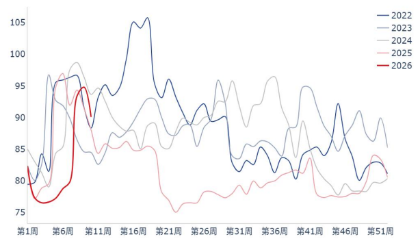
热轧卷板钢厂库存
