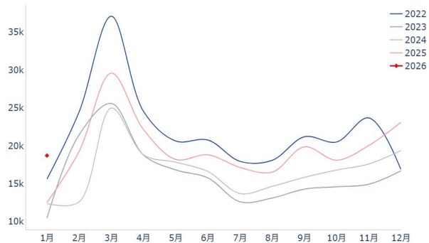
挖掘机销量
