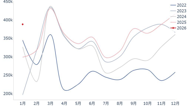
商用车产量
