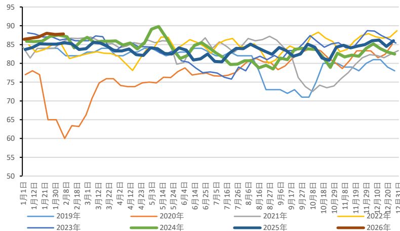
样本企业烧碱开工率
