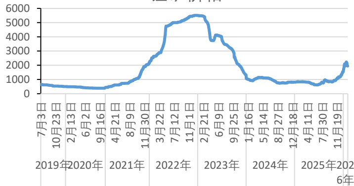
锂矿价格
