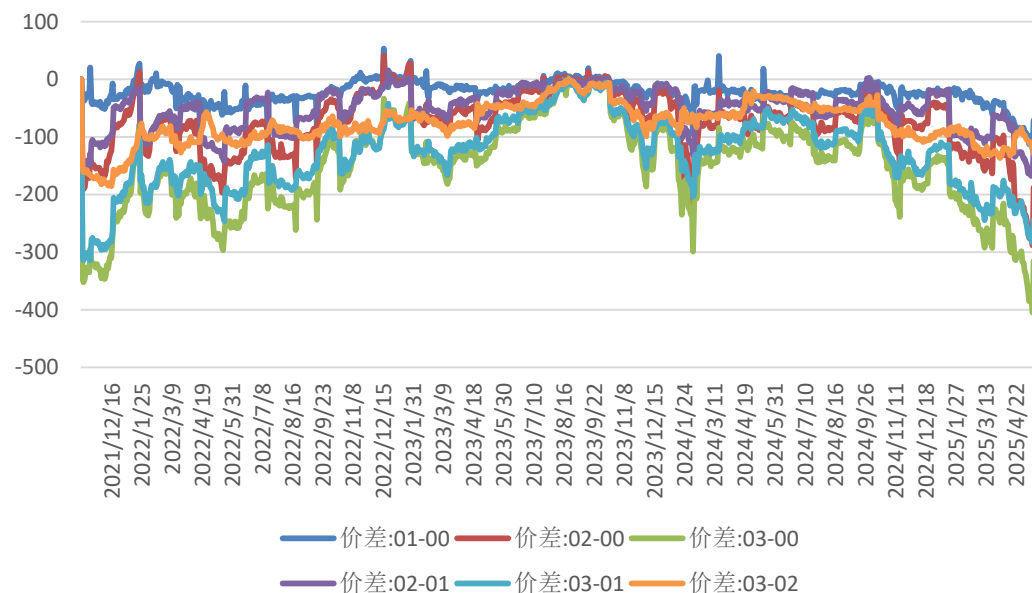
中证500价差
