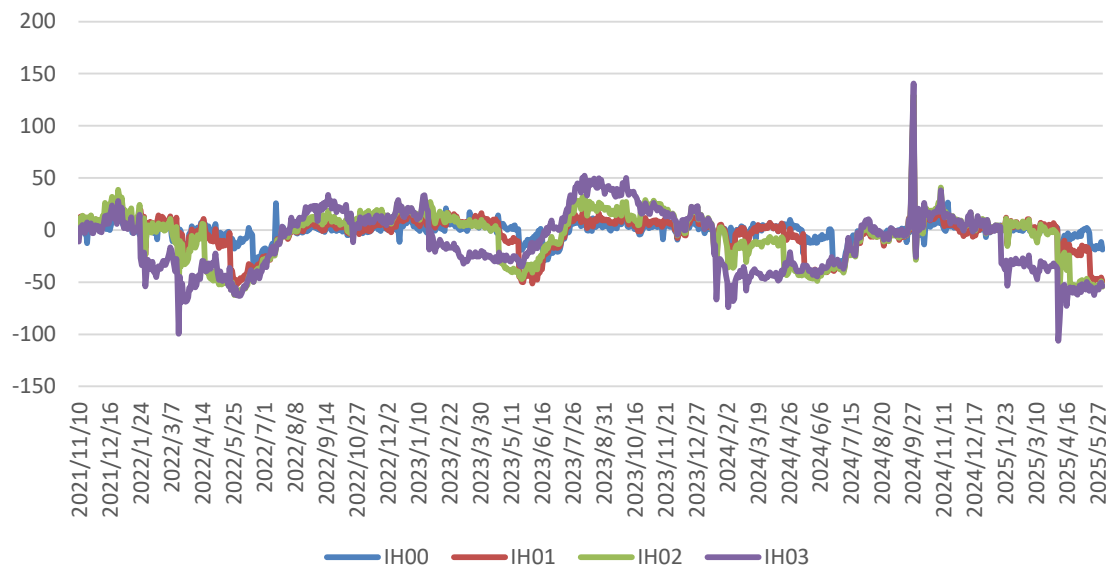
上证50基差
