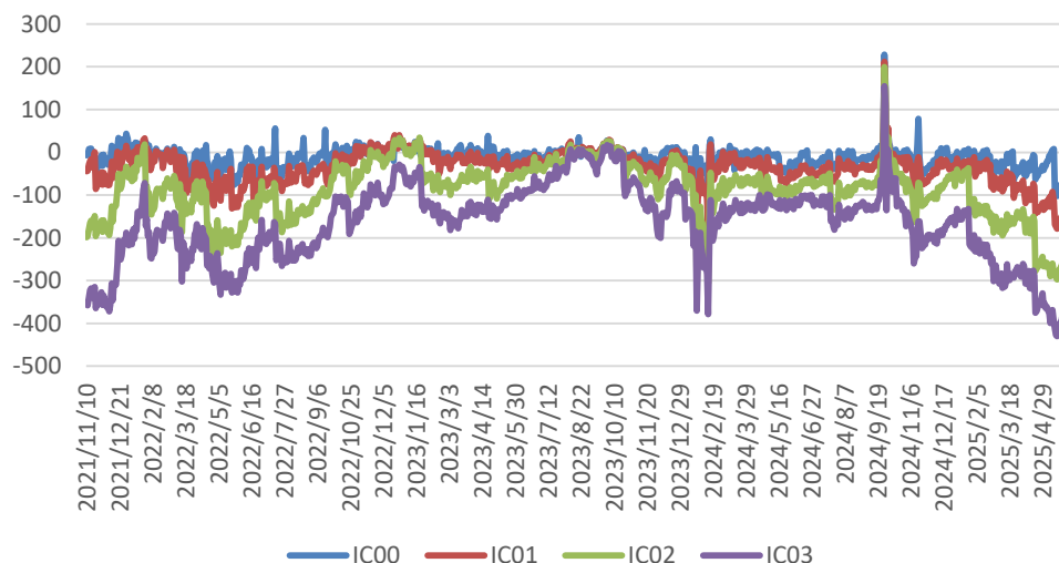
中证500基差
