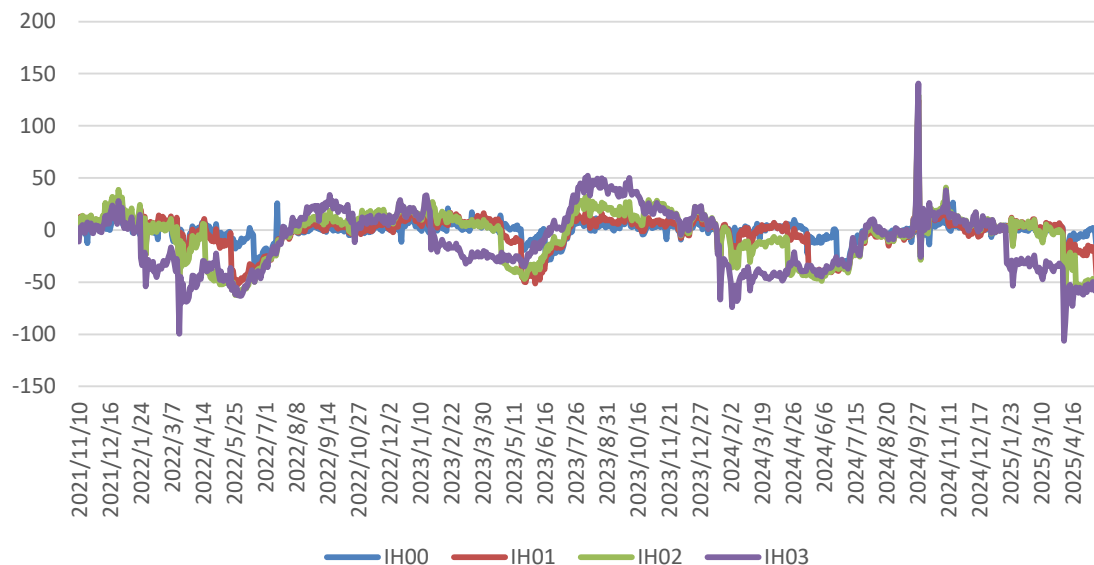
上证50基差
