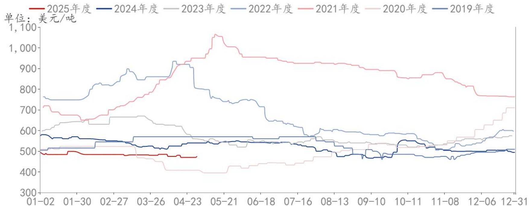
热轧板卷：进口：CFR价：东南亚（日）
