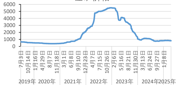
锂矿价格
