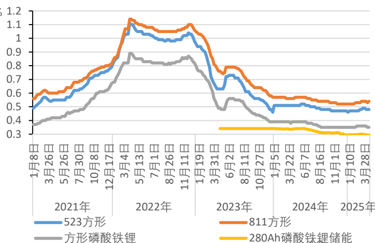
电芯成本
