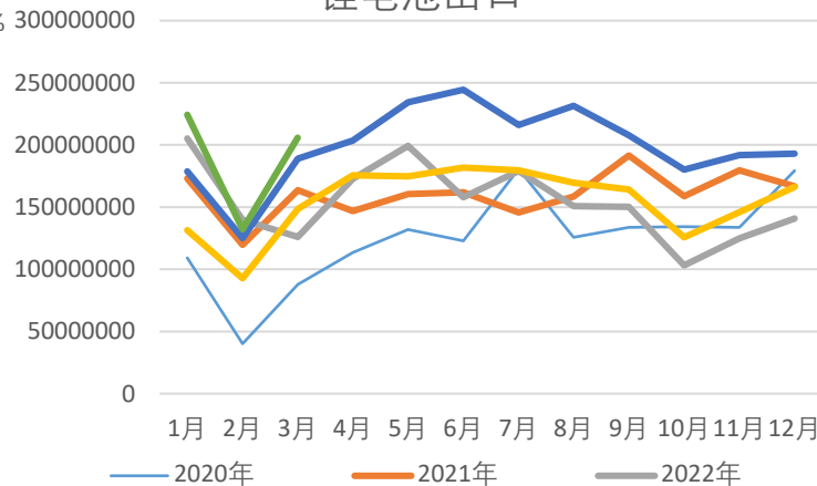
锂电池出口
