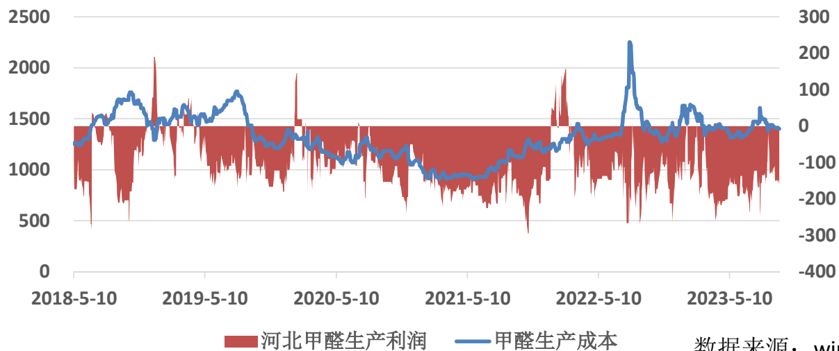
甲醛生产成本和利润
