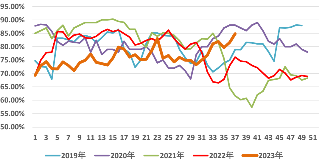
MTO/MTP装置负荷
