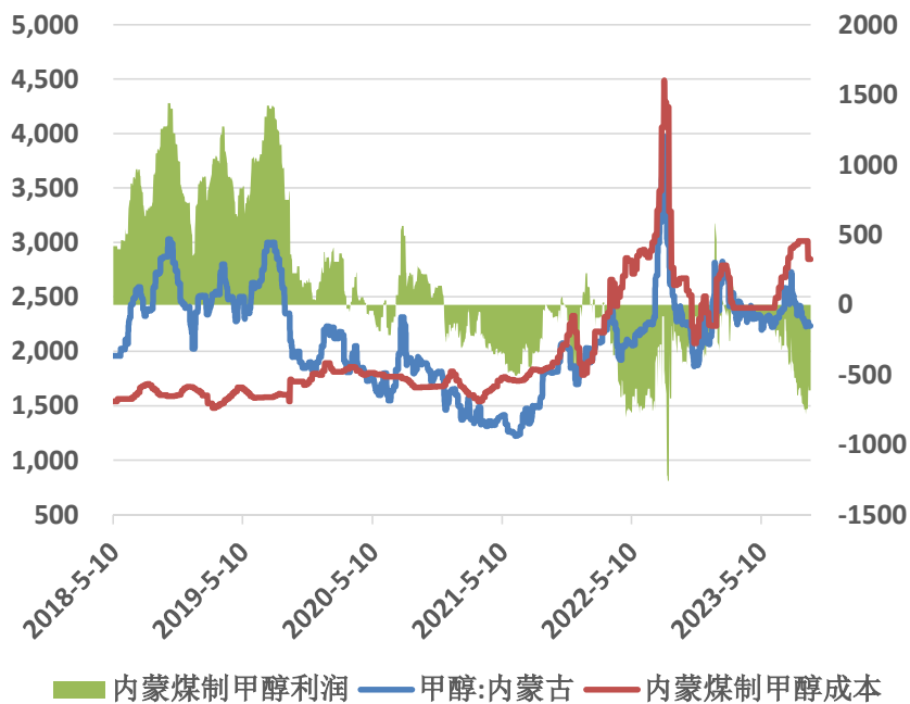
内蒙煤制甲醇成本及利润
